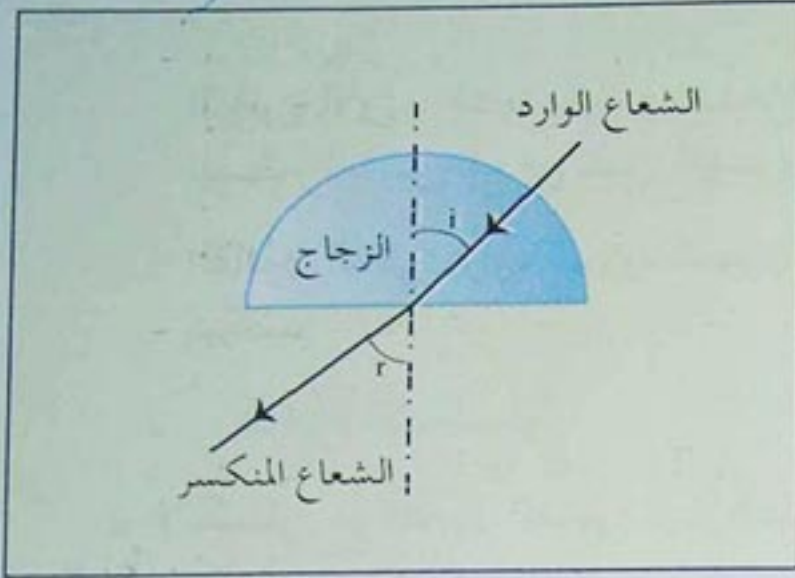
الشكل 4 : منظر علوي لمخطط التجربة
