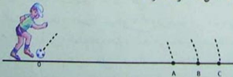
الشكل 1: كرة مقذوفة
