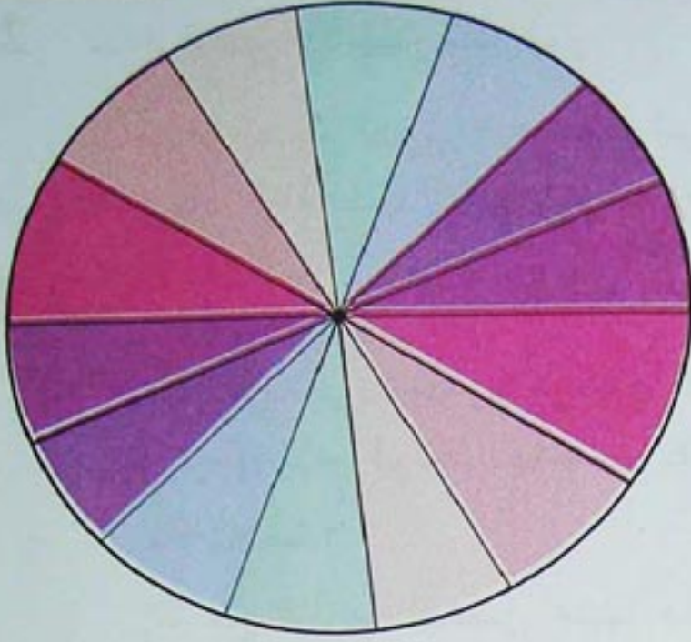
الشكل 6 : قرص نيوتن
