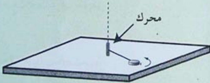
الشكل 4 : جسم يدور فوق طاولة
