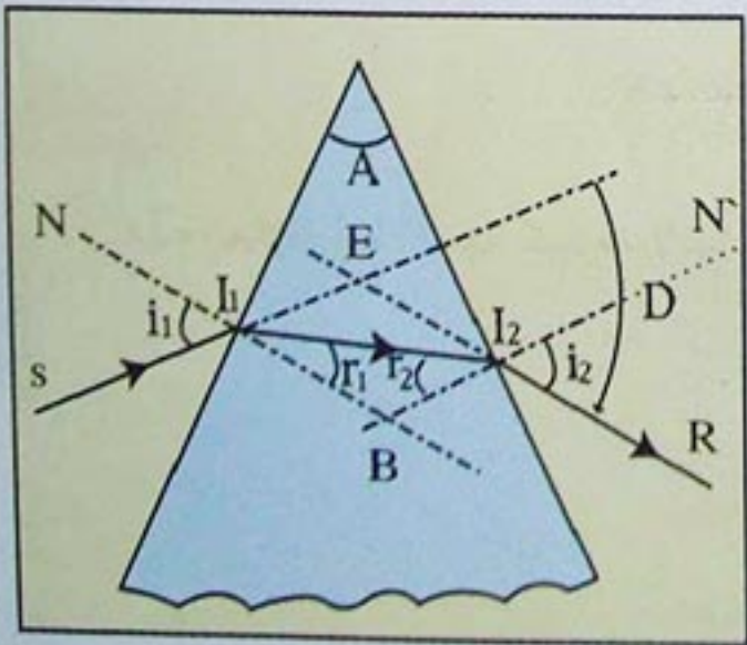
الشكل 6 : مخطط مسير الشعاع الضوئي والزاويا المميزة
